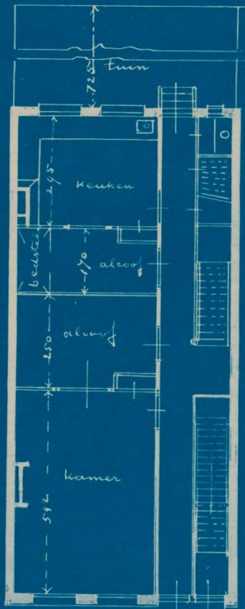
Begane grond Bestaande toestand
