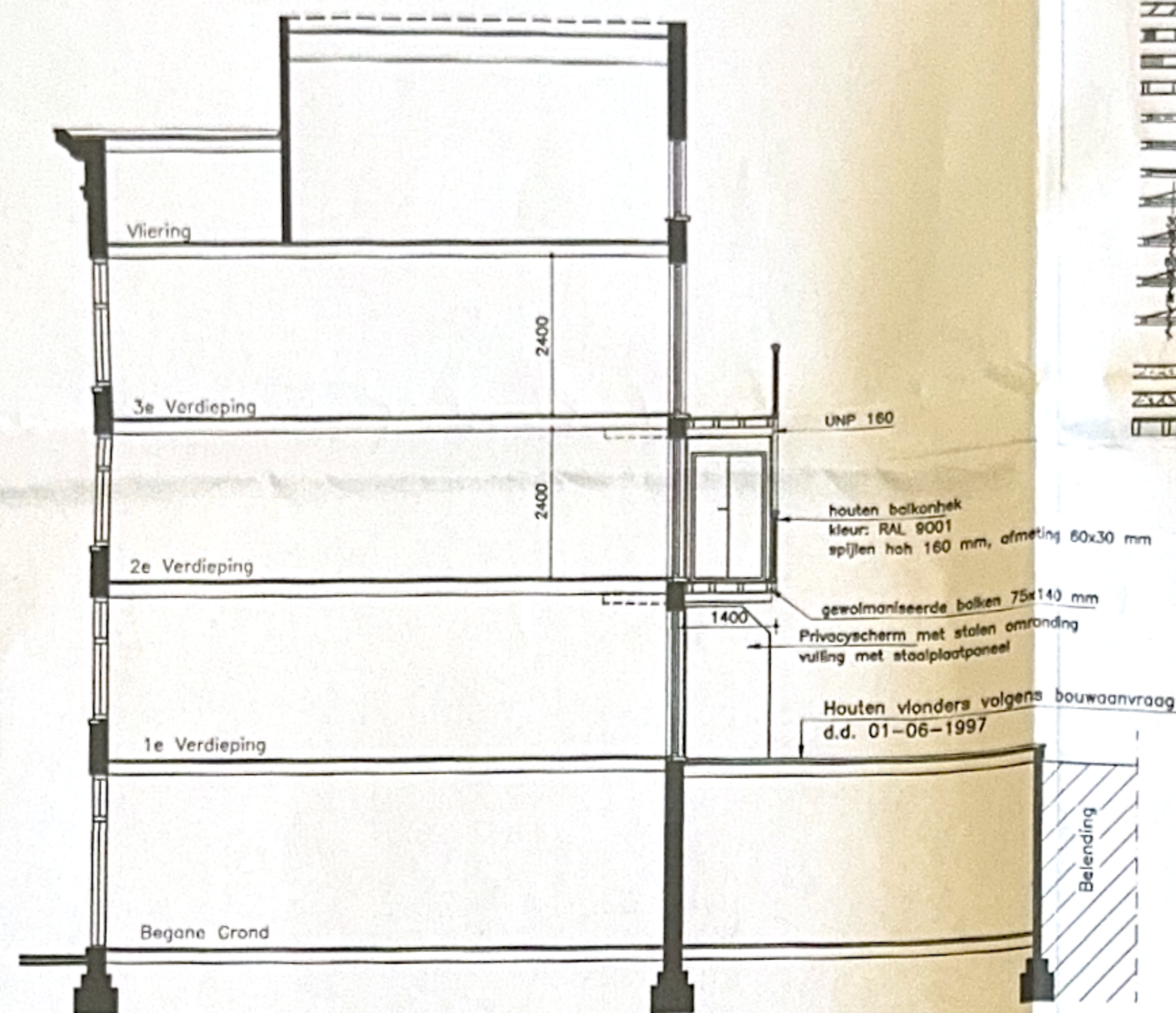
Doorsnede A-A
