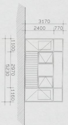
voorgevel (bestaand)
